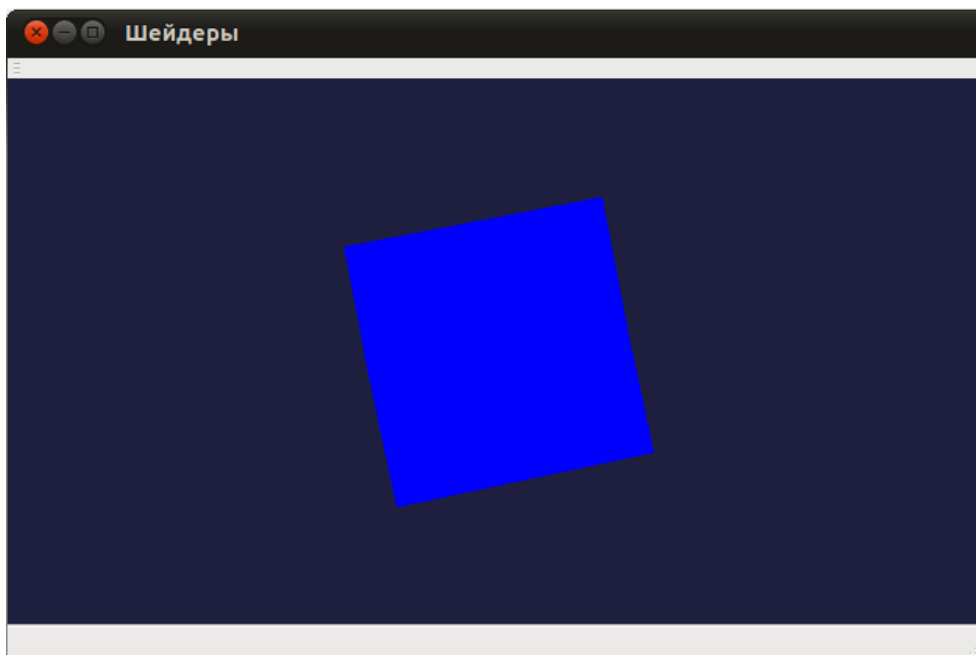
Рис. 4. Программа shader-demo
