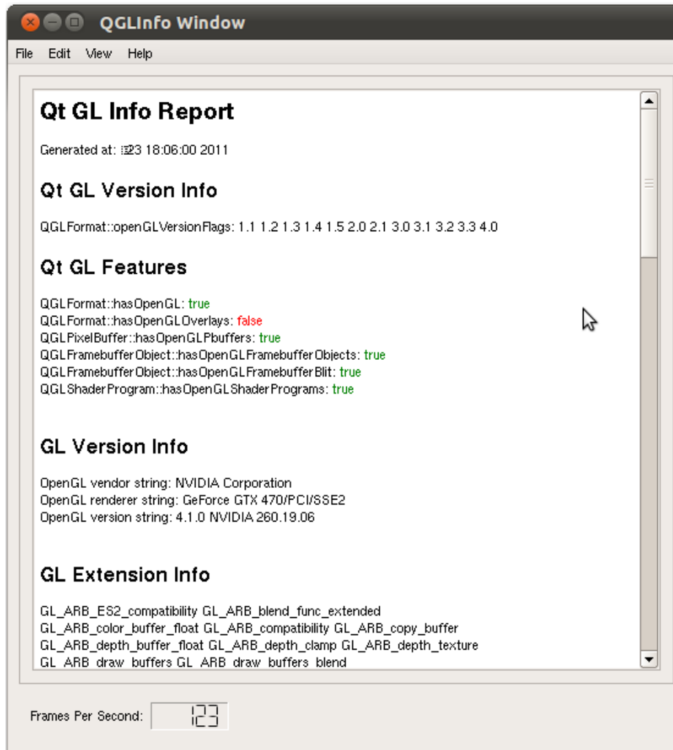
Рис. 7. Окно программы qglinfo
